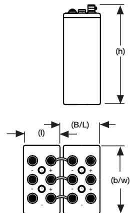
16 OPzS 2000 bis 18 OPzS 2250
