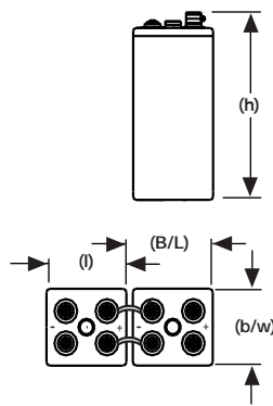
8 OPzS 800 bis 14 OPzS 1750
