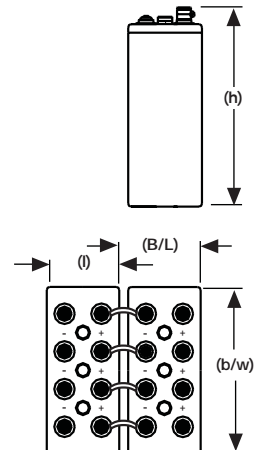
20 OPzS 2500 bis 24 OPzS 3000
